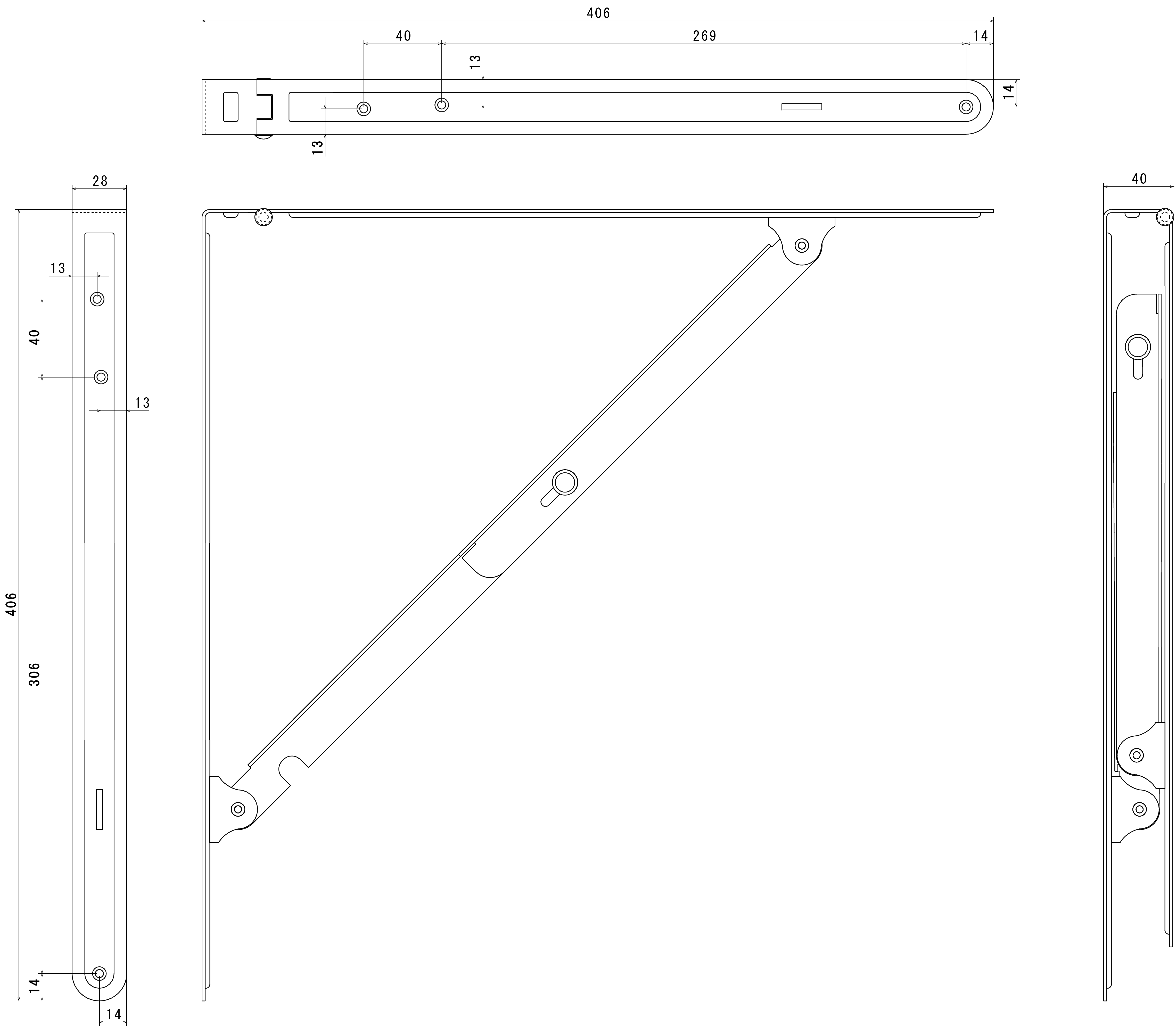
400mm 寸法図 【S=1/1】
